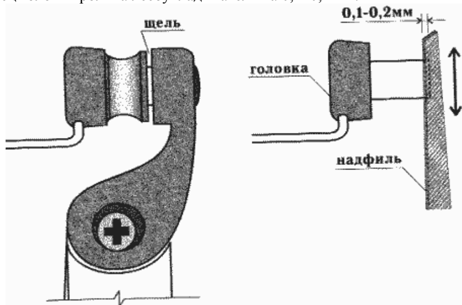
Рис. 6. Щель между роликом и рычагом лесокладывателя
