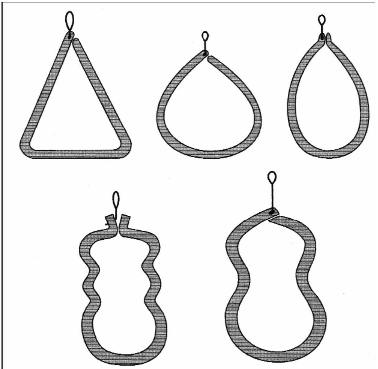
Рис. 74. Отцепы для глубоководных воблеров (диаметр прутка 8–12 мм)
